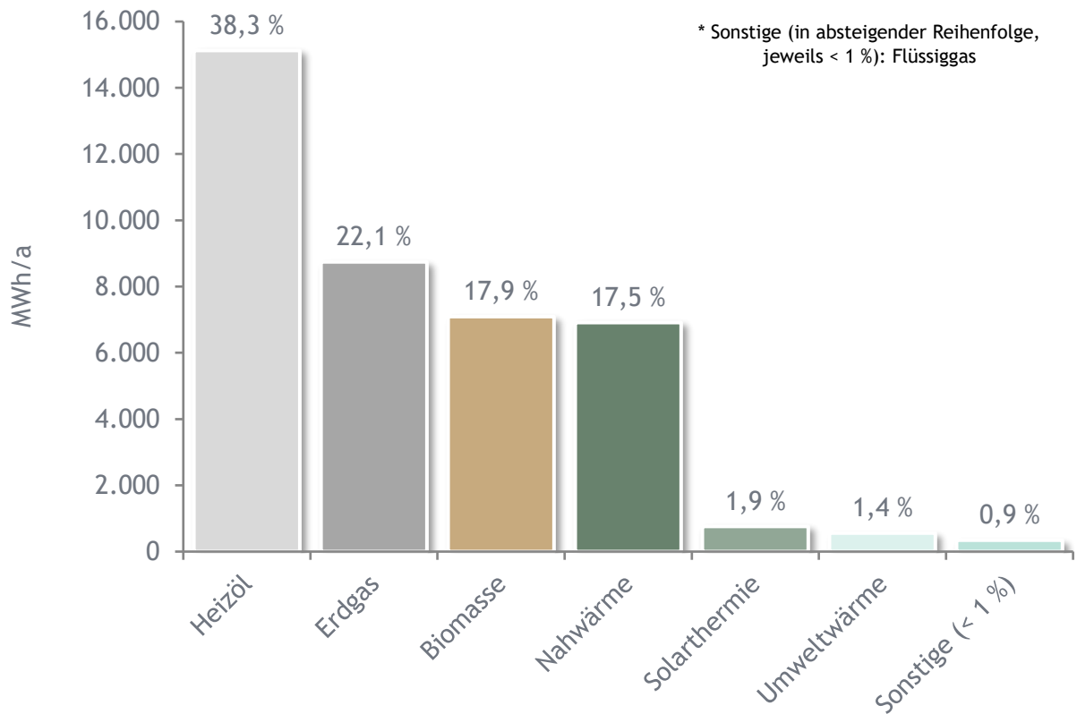
Abbildung 9: Wärmeverbrauch nach Energieträgern, eigene Darstellung
