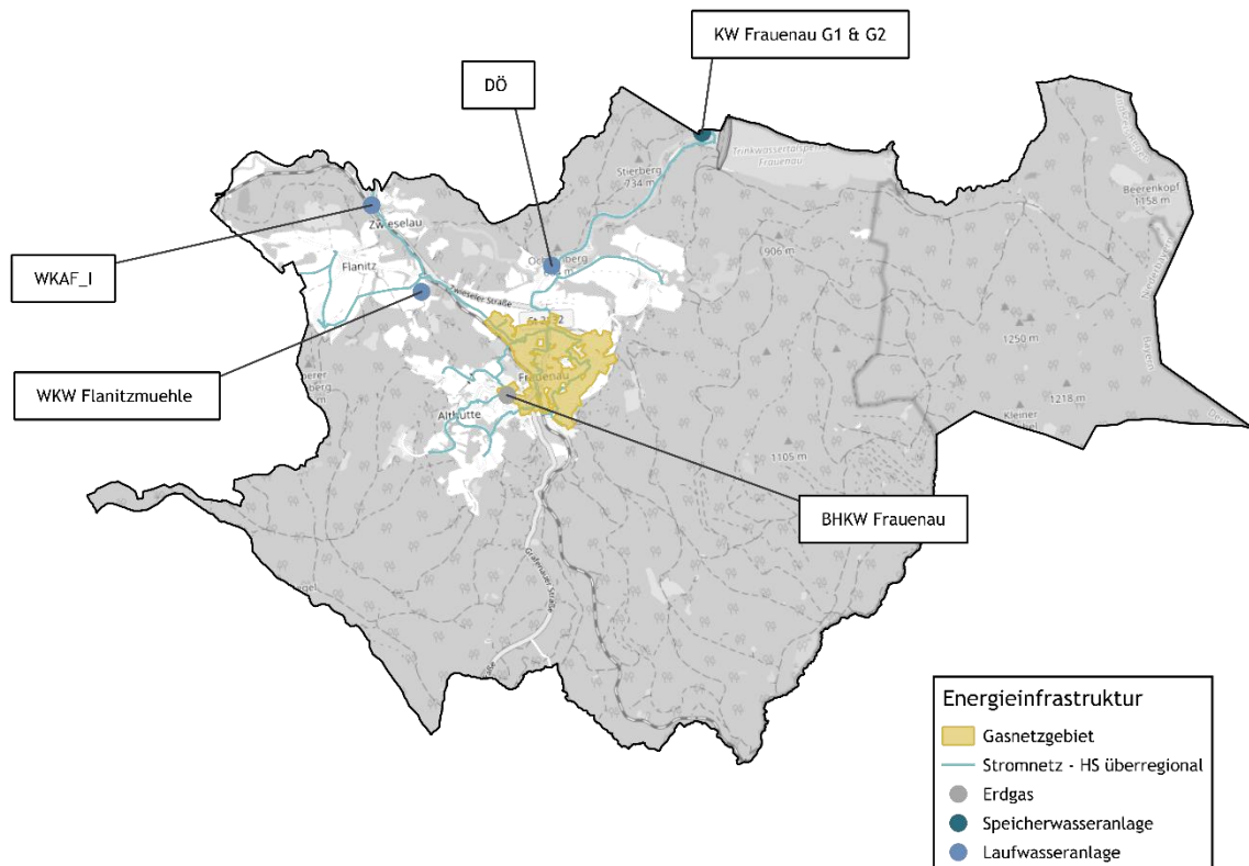
Abbildung 1: Energieversorgung in Frauenau: Standorte der Wasserkraftwerke und Erdgas-BHKW sowie der Verlauf des Strom- und Gasnetzes, eigene Darstellung
