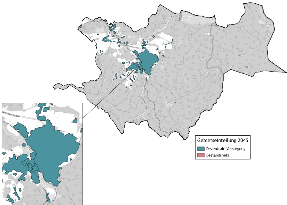
Abbildung 33: Einteilung der Wärmeversorgungsgebiete in Frauenau im Zieljahr 2045, eigene Darstellung
