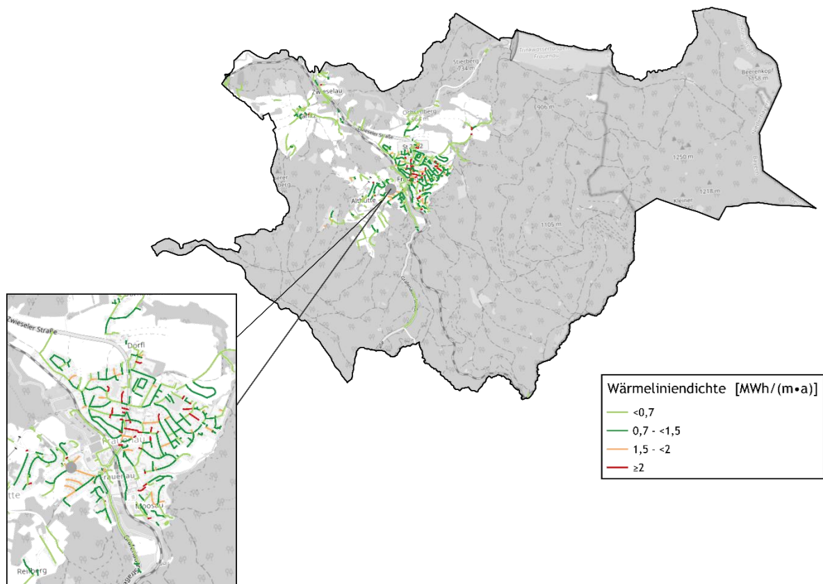
Abbildung 18: Wärmelinienendichten in Frauenau, eigene Darstellung
