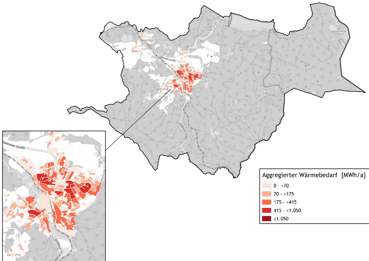
Abbildung 17: Aggregierter Wärmebedarf auf Baublockebene in Frauenau, eigene Darstellung
