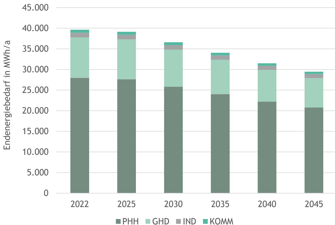
Abbildung 35: Entwicklung des Wärmebedarfs nach Sektoren für die Jahre 2025, 2030, 2035, 2040 und 2045, eigene Darstellung
