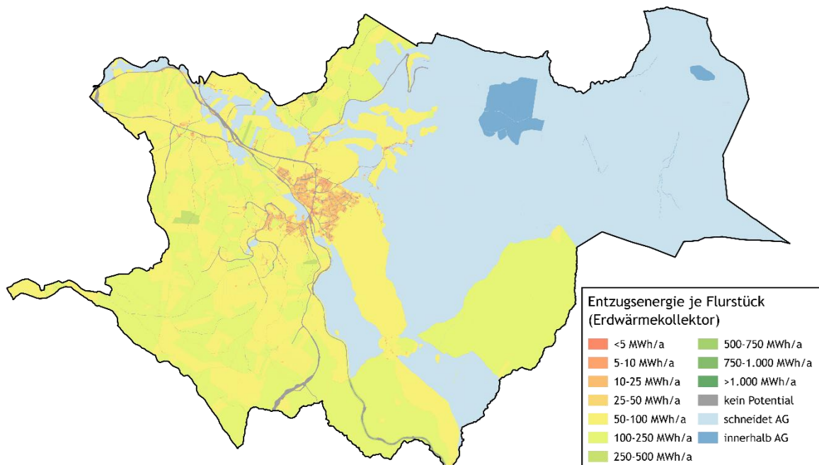
Abbildung 22: Oberflächennahe Geothermie: Entzugsleistungen von Erdwärmekollektoren in Frauenau [8]
