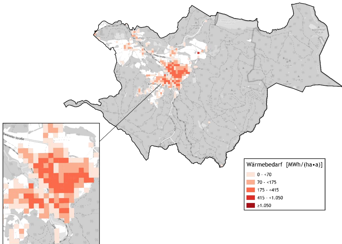
Abbildung 16: Wärmebedarf nach Hektarraster in Frauenau, eigene Darstellung
