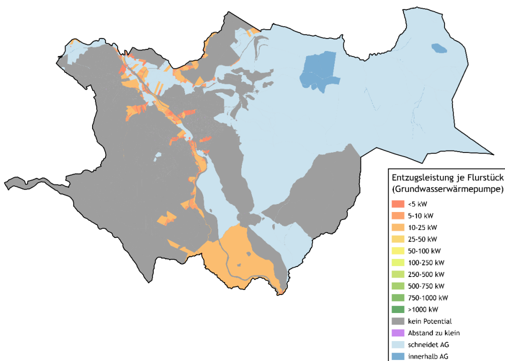
Abbildung 24: Oberflächennaher Geothermie: Entzugsleistungen von Grundwasserwärmepumpen in Frauenau [8]
