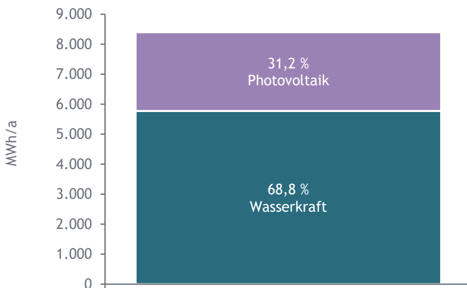
Abbildung 14: Energiequellenverteilung des erneuerbaren Stroms, eigene Darstellung
