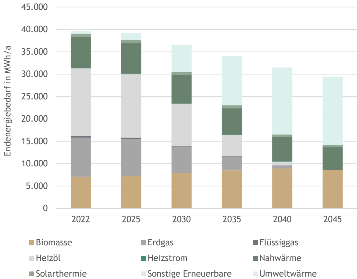
Abbildung 36: Entwicklung des Wärmebedarfs nach Energieträgern für die Jahre 2025, 2030, 2035, 2040 und 2045, eigene Darstellung
