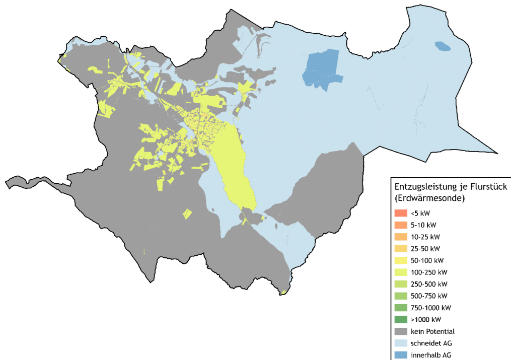
Abbildung 23: Oberflächennaher Geothermie: Entzugsleistungen von Erdwärmesonden in Frauenau [8]
