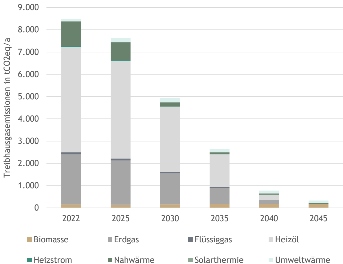
Abbildung 37: Entwicklung der THG-Emissionen aus dem prognostizierten Strom- und Wärmebedarf für die Jahre 2025, 2030, 2035, 2040 und 2045, eigene Darstellung
