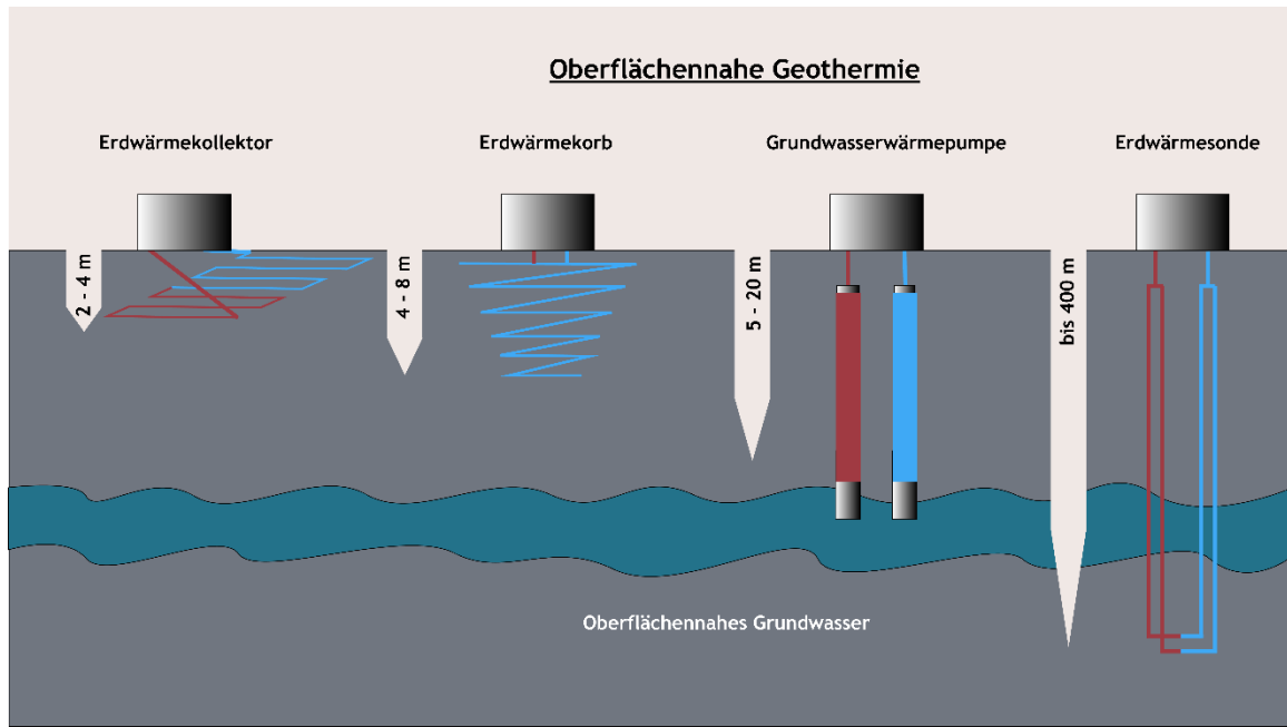
Abbildung 21: Funktionsprinzipien und Technologien der oberflächennahen Geothermie, eigene Darstellung
