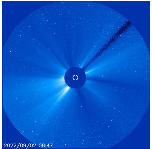
Bild 8 C3-Koronograph
