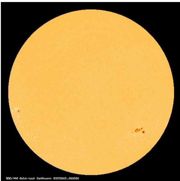
Bild 5 Visuelle Sonne
