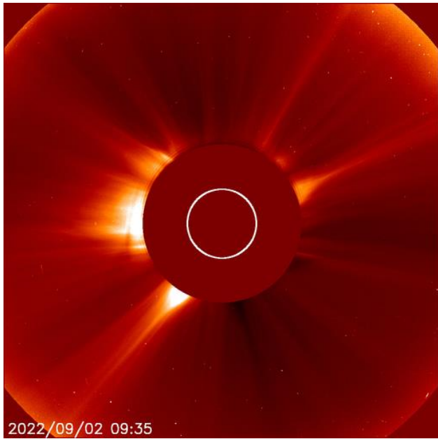
Bild 7 C2- Koronograph
