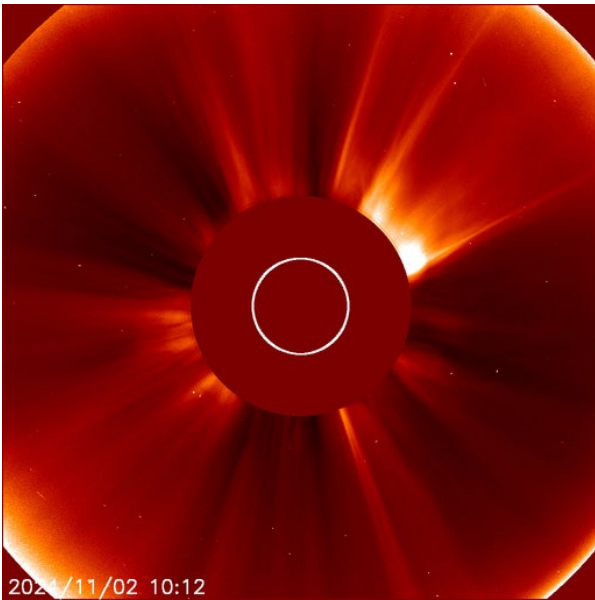
Bild 7 C2- Koronograph
