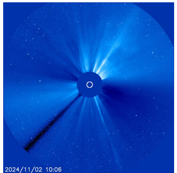
Bild 8 C3-Koronograph
