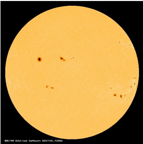
Bild 5 Visuelle Sonne
